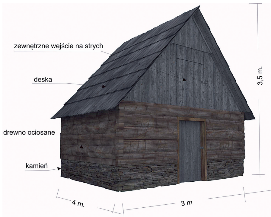
Ryc. 4. Schemat konstrukcyjno-architektoniczny szopy drewniano-kamiennej Fig. 4. Construction scheme of architecture of a wooden-stone shed
