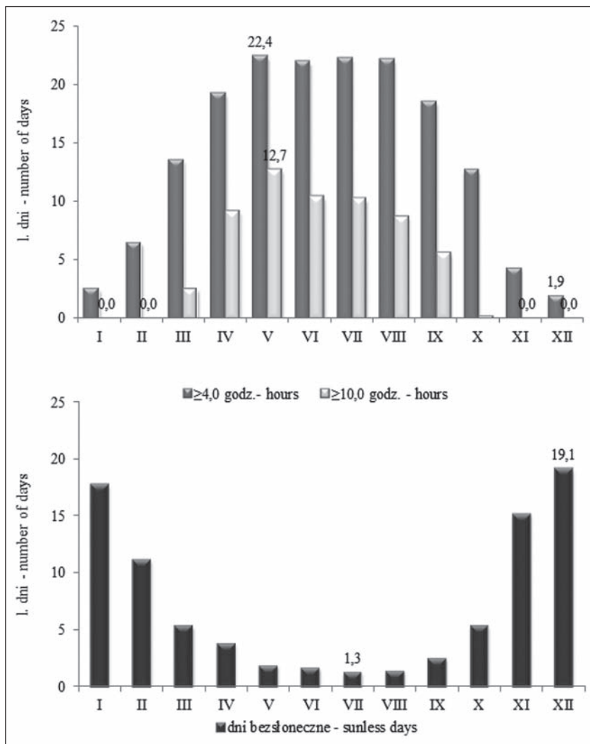
Ryc. 7. Przebieg roczny liczby dni o określonej wielkości usłonecznienia w Koniczynce w latach 1999–2013
