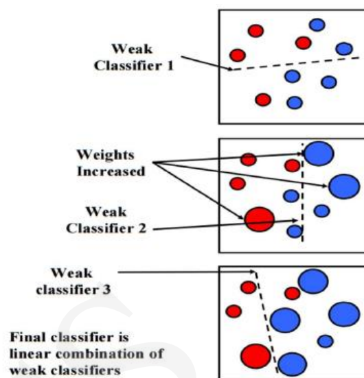
Fig. 3 AdaBoost[4]
